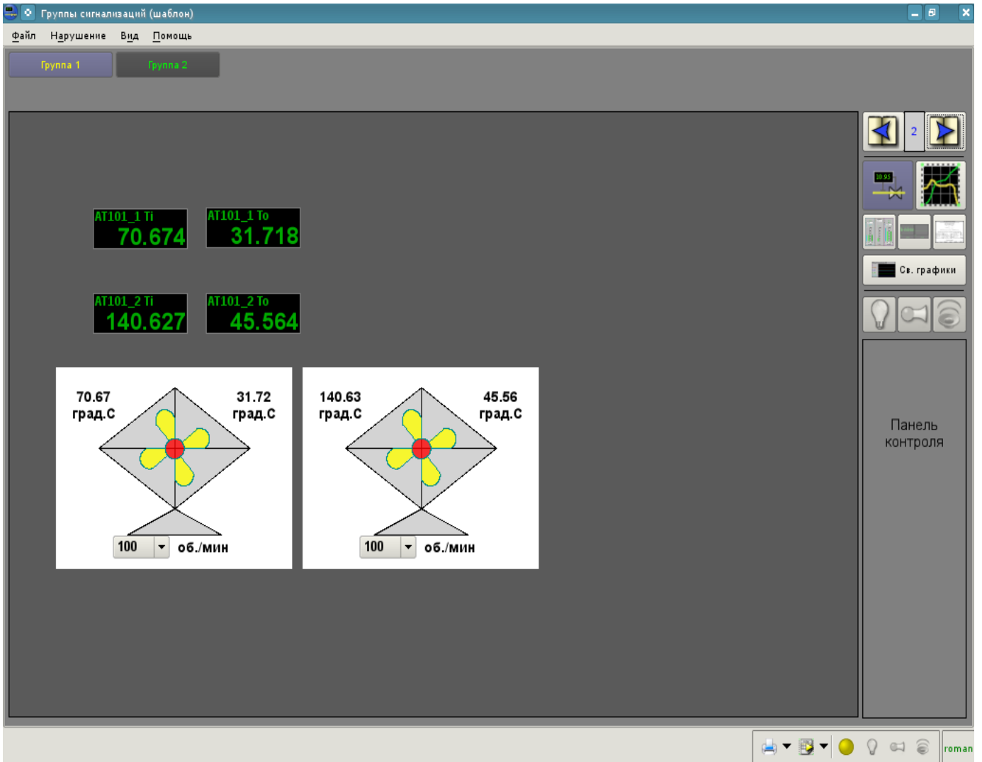
Рис. 5.3.3.3. Результирующая мнемосхема.
