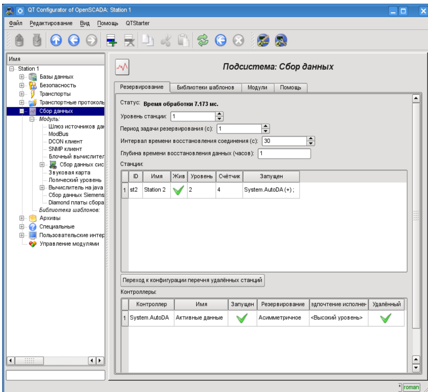
Рис. 4.5б. Вкладка "Резервирование" подсистемы "Сбор данных".
