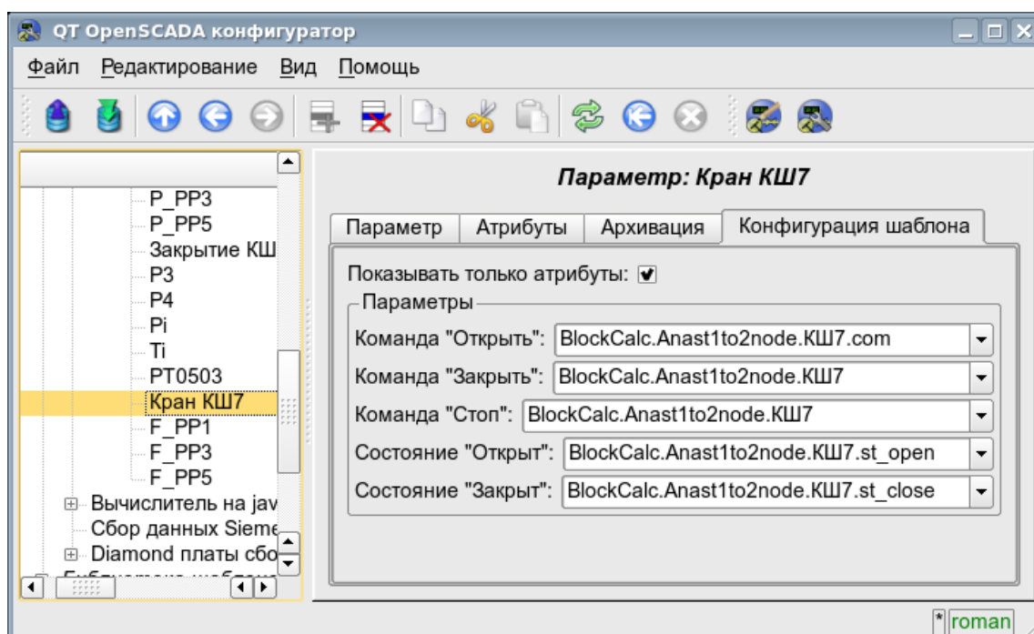
Рис.4. Вкладка конфигурации шаблона параметра. Показывать только атрибуты
