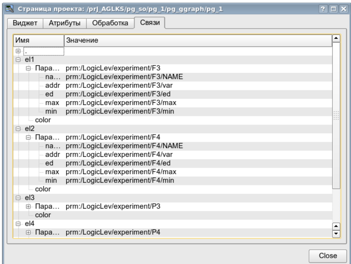
Рис.7. Вкладка связей диалога редактирования свойств визуального элемента.
