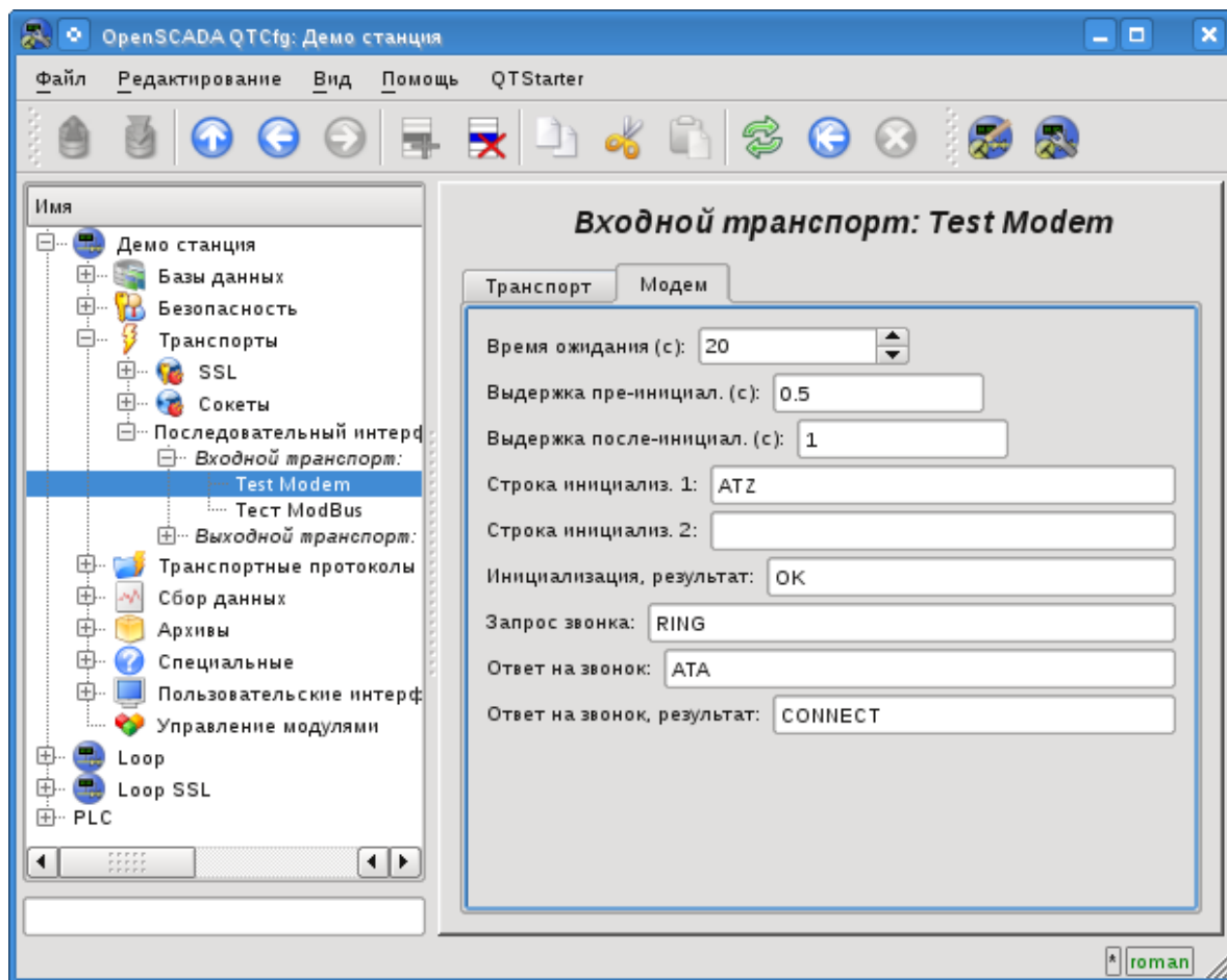
Рис.2. Вкладка "Модем" конфигурации модема входящего последовательного интерфейса.
