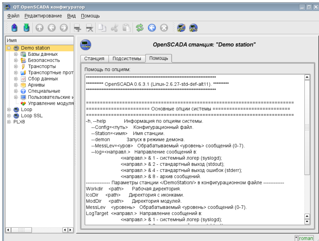
Рис. 4.10а. Вкладка "Помощь" компонента OpenSCADA.
