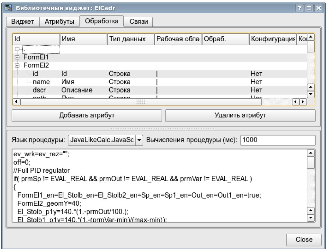
Рис.6. Вкладка обработки диалога редактирования свойств визуального элемента.
