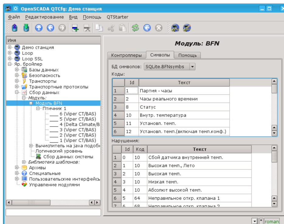
Рис.1. Вкладка конфигурации символов сигналов и нарушений.
