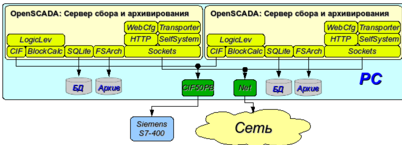
Рис. 3.3. Дублированное серверное подключение на одном сервере.
