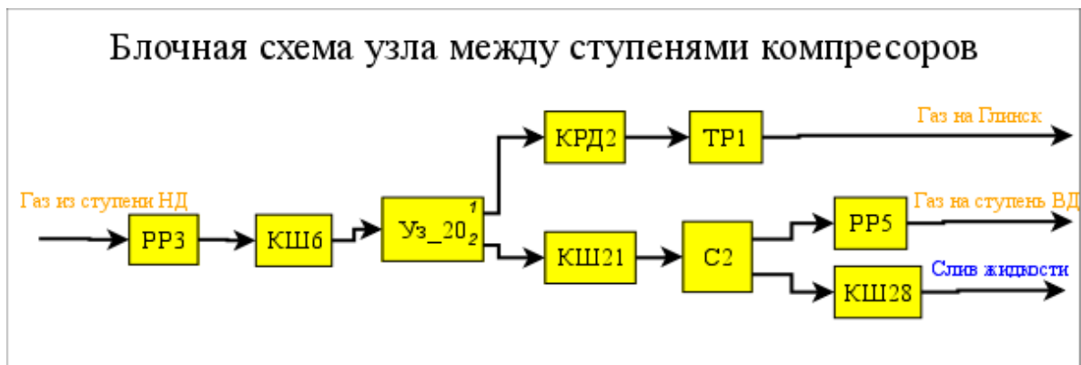
Рис. 1. Общие связи между блоками блочной схемы
