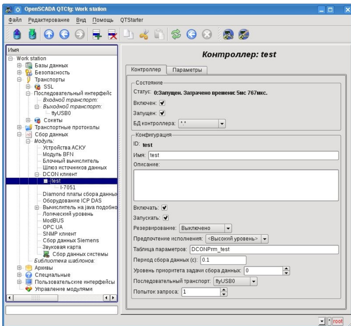
Рис.1. Вкладка конфигурации контроллера.
