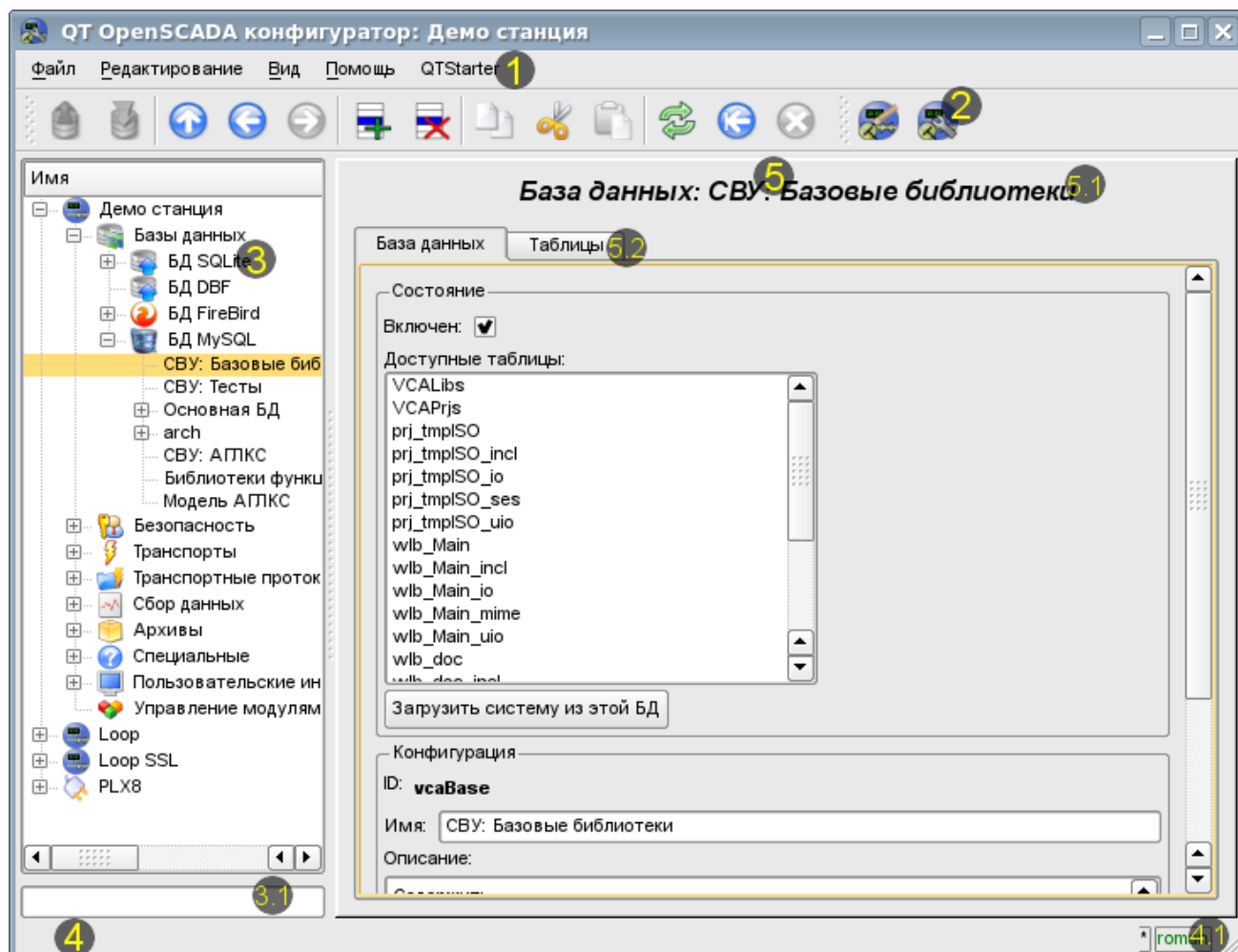
Рис. 1. Рабочее окно конфигулятора
