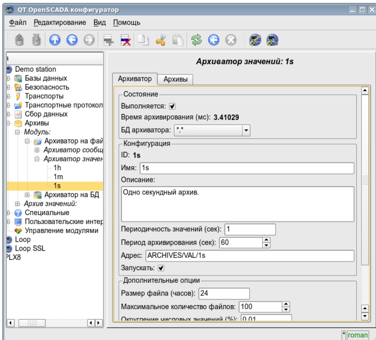
Рис. 4.6j. Главная вкладка конфигурации архиватора значений подсистемы "Архивы".
