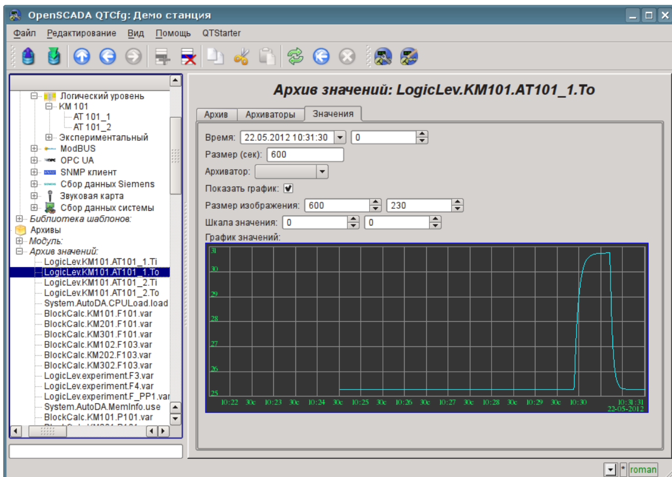
Рис. 4.4.3. Вкладка "Значения" страницы объекта архива атрибута "To" параметра AT101_1.
