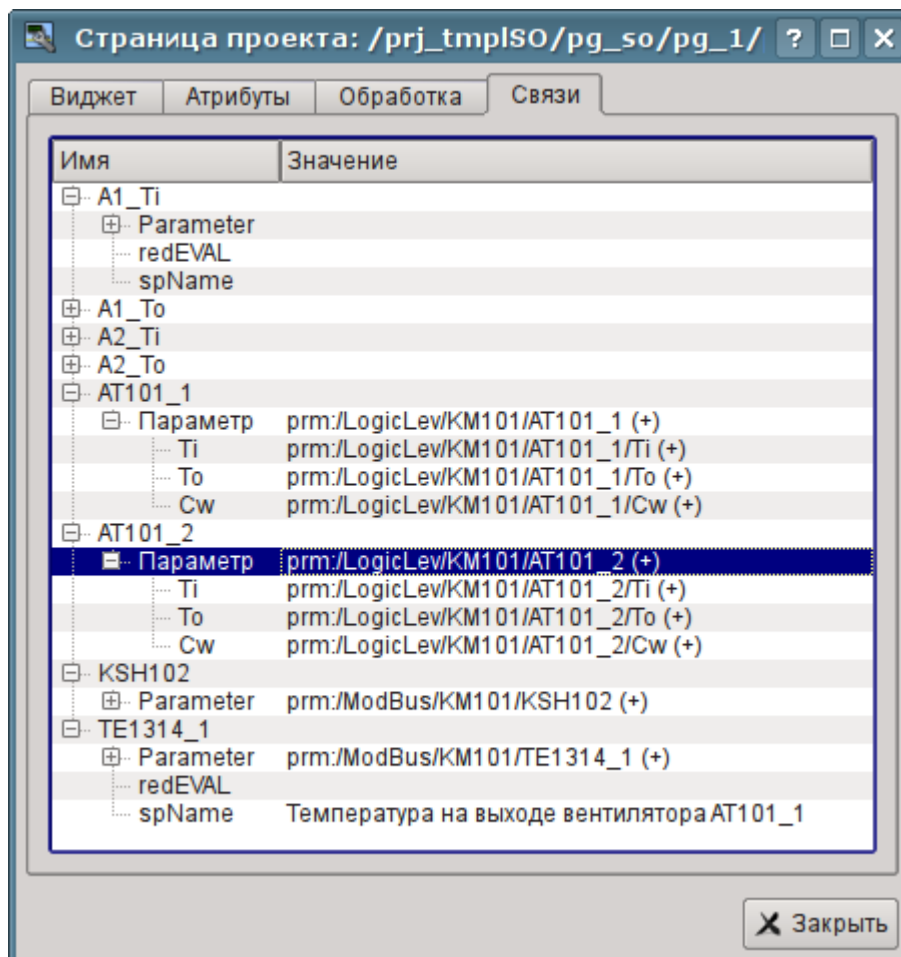
Рис. 5.3.3.2. Вкладка "Связи" диалога редактирования свойств мнемосхемы.
