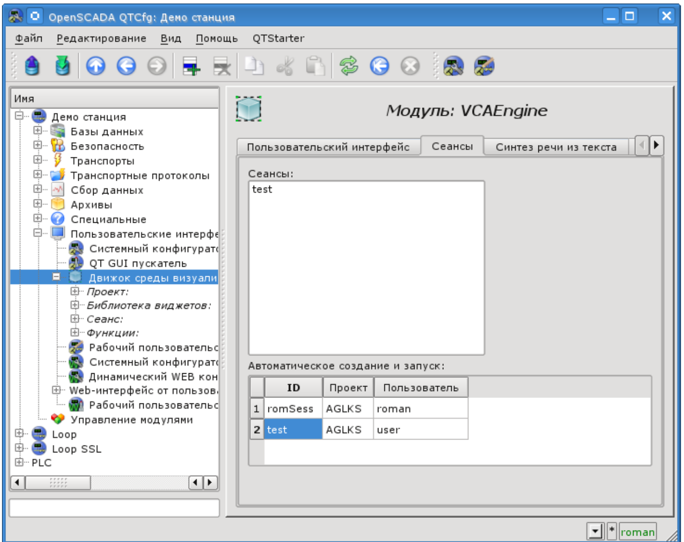
Рис.4.2 Вкладка "Сессии" конфигурационной страницы модуля.
