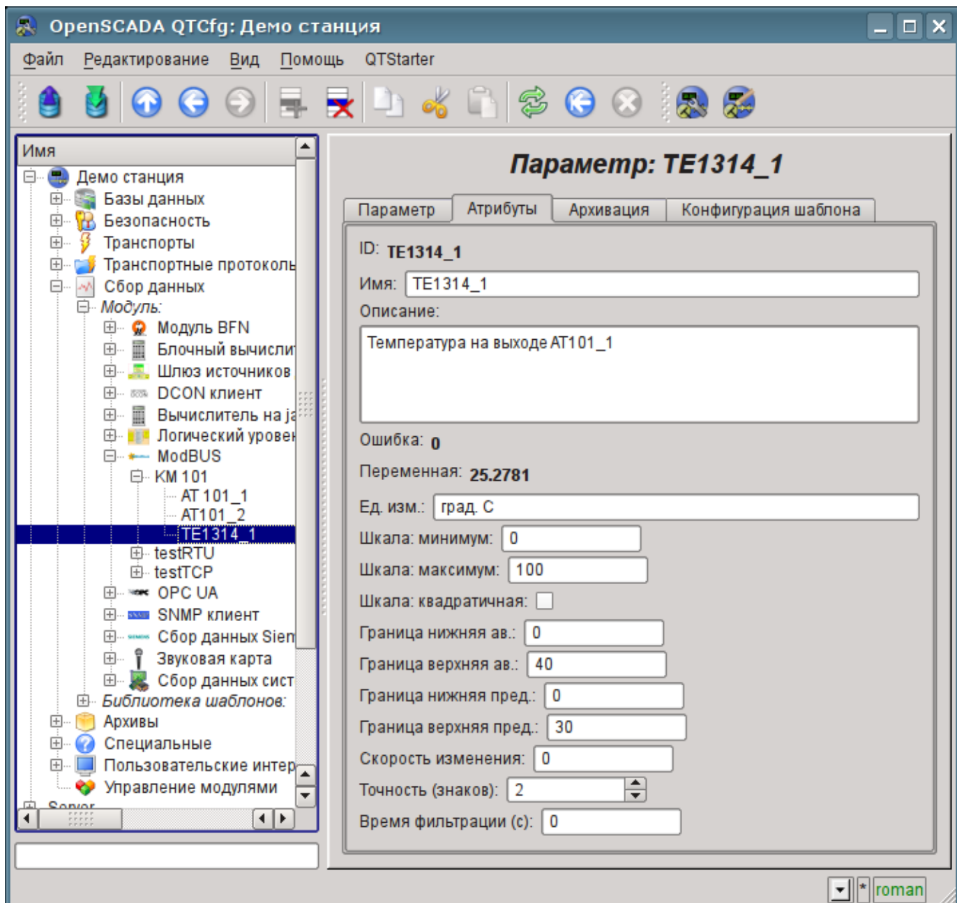
Рис. 4.3.3. Страница атрибутов параметра "TE1314_1", модуля "ModBus".
