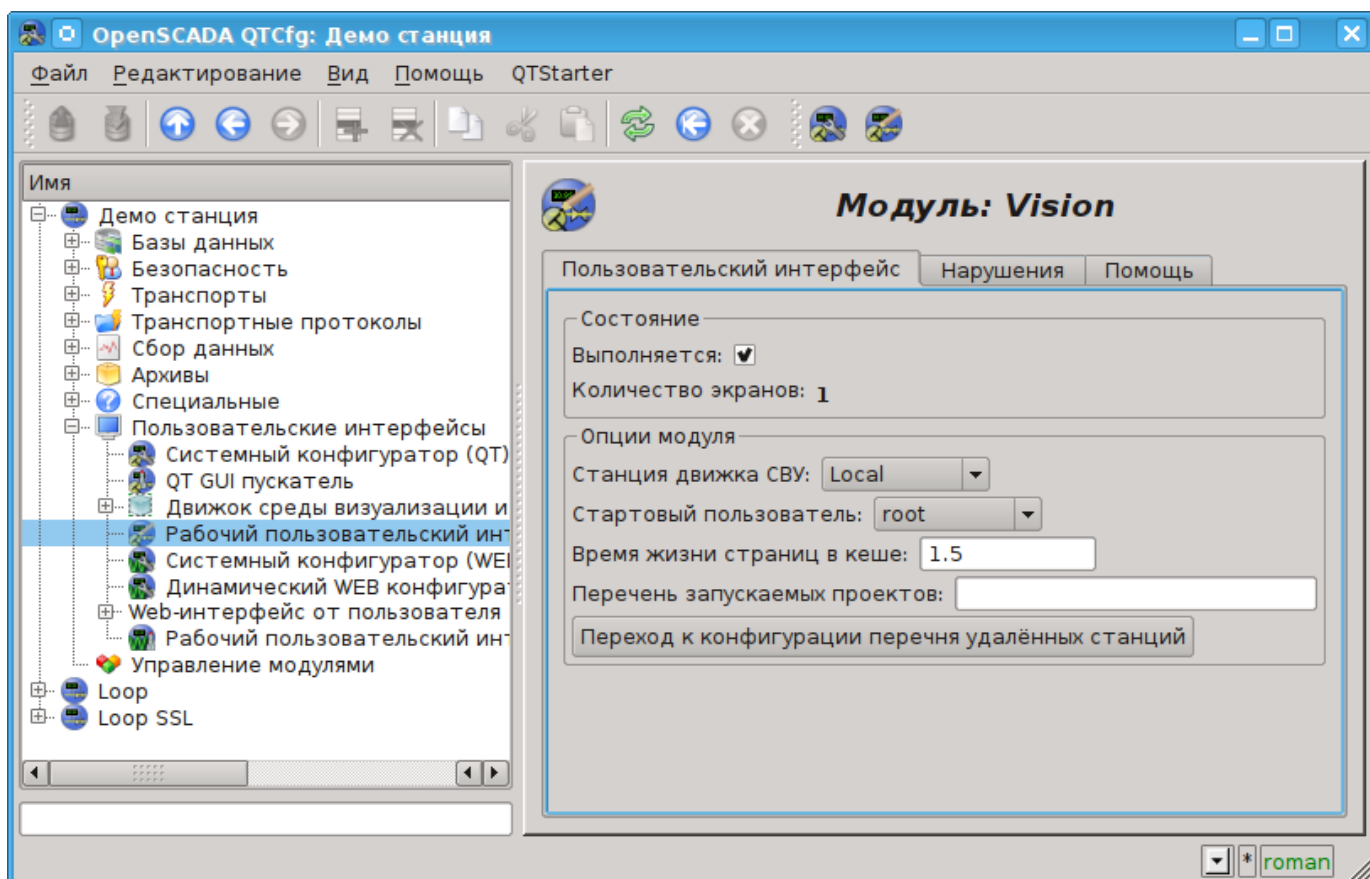
Рис.6.a. Страница конфигурации модуля.
