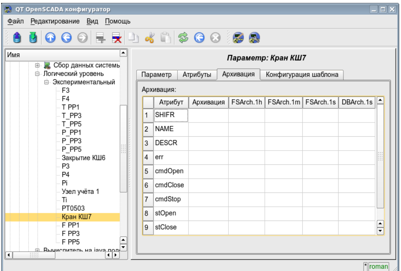
Рис. 4.5т. Вкладка "Архивация" параметра контроллера подсистемы "Сбор данных".
