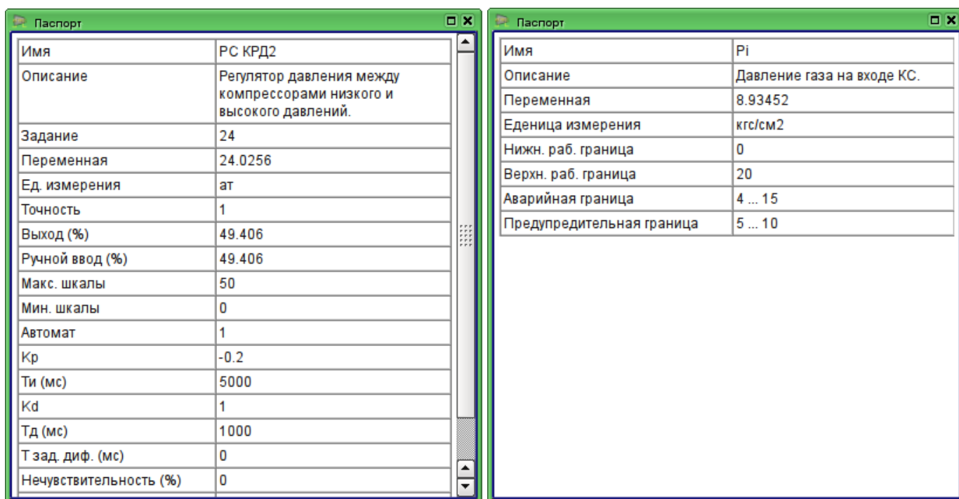
Рис.23. Виджет "Паспорт" в режиме исполнения.
