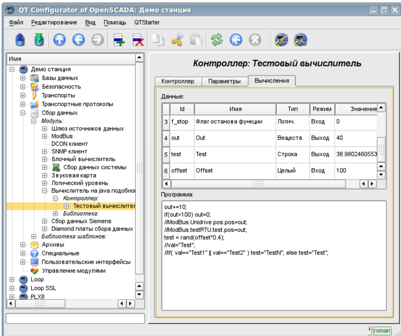
Рис.3. Вкладка «Вычисления» контроллера.
