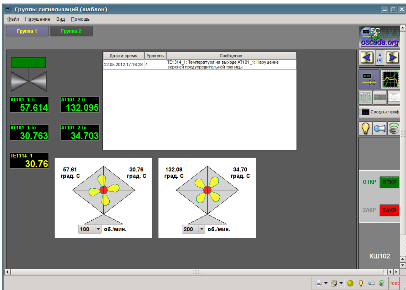
Рис. 5.3.3.3. Результирующая мнемосхема.
