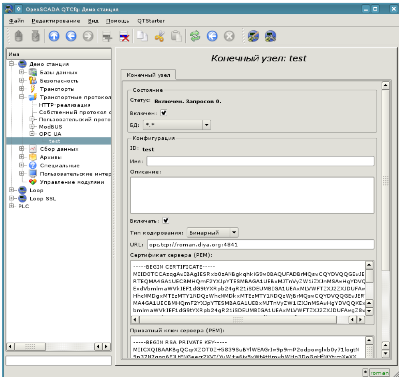
Рис.2. Главная вкладка страницы конечного узла.
