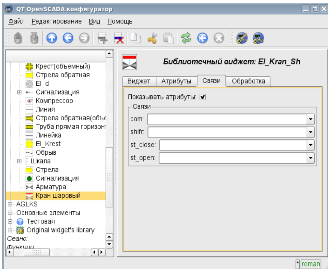
Рис. 3.7.с Вкладка "Связи" страницы конфигурации виджета с индивидуальным назначением атрибутов.
