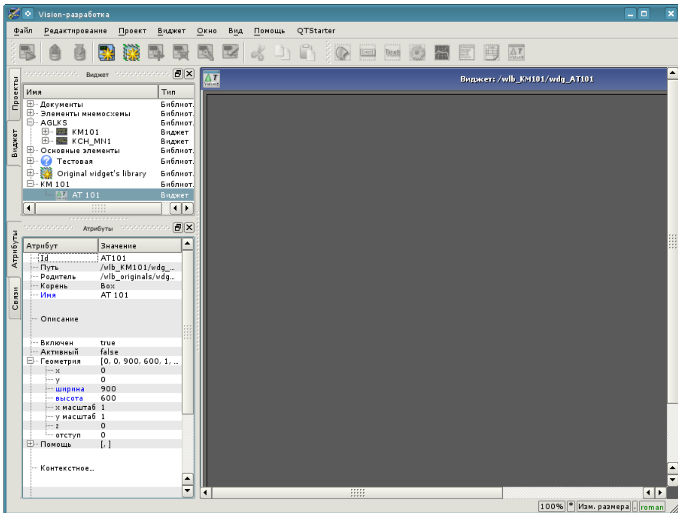
Рис. 5.2.3. Вид нового кадра и установленных атрибутов для мнемосхемы.
