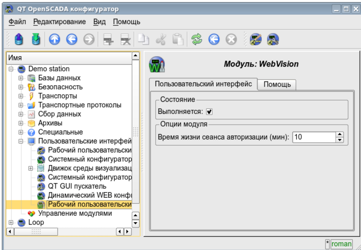
Рис.11. Страница конфигурации модуля.
