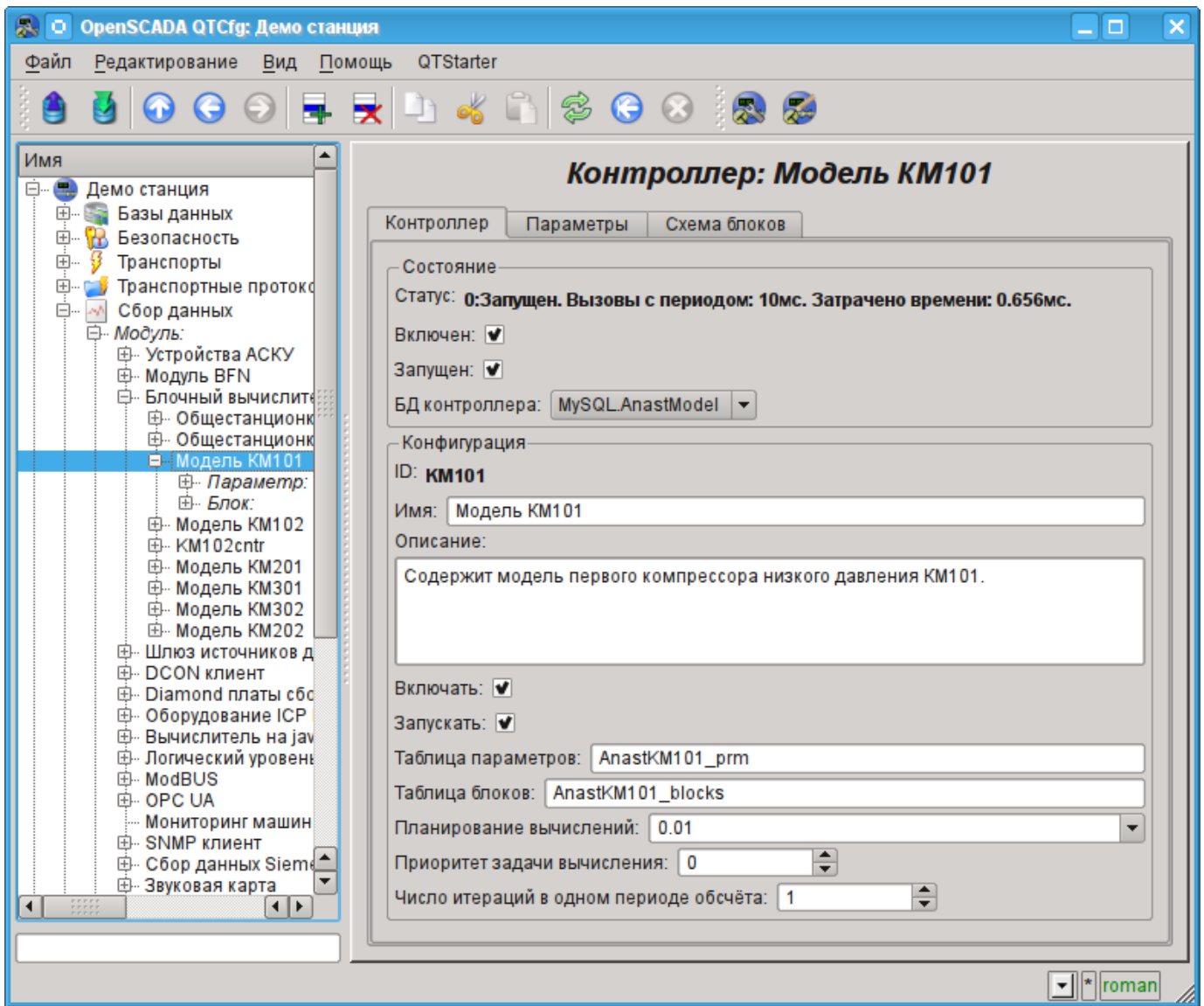
Рис. 3. Вкладка конфигурации контроллера.
