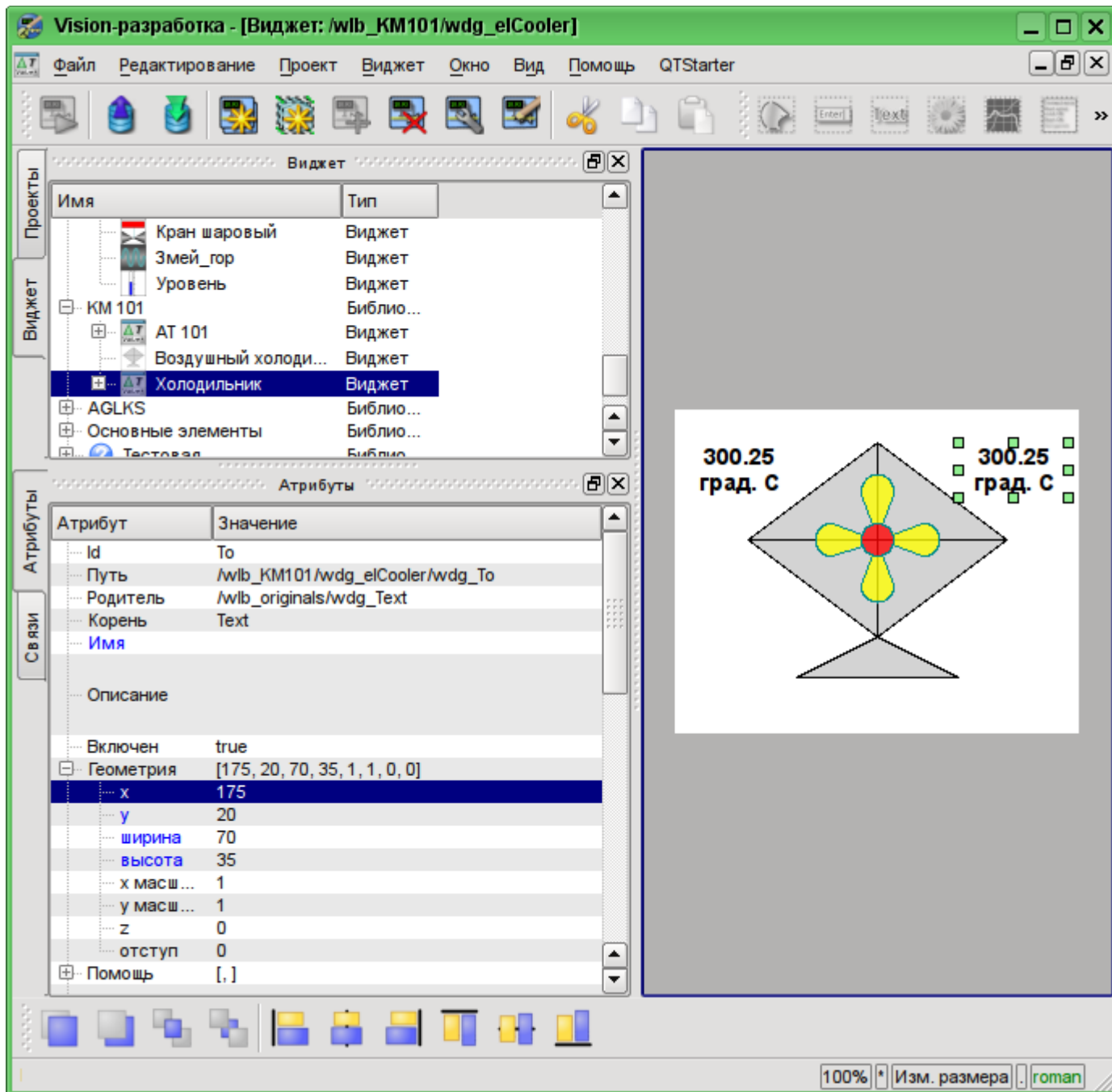
Рис. 5.3.2.10. Виджет "To".
